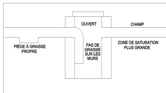
Les solides sont dégradés et liquéfiés pour ensuite être absorbés par le champ d'infiltration.
